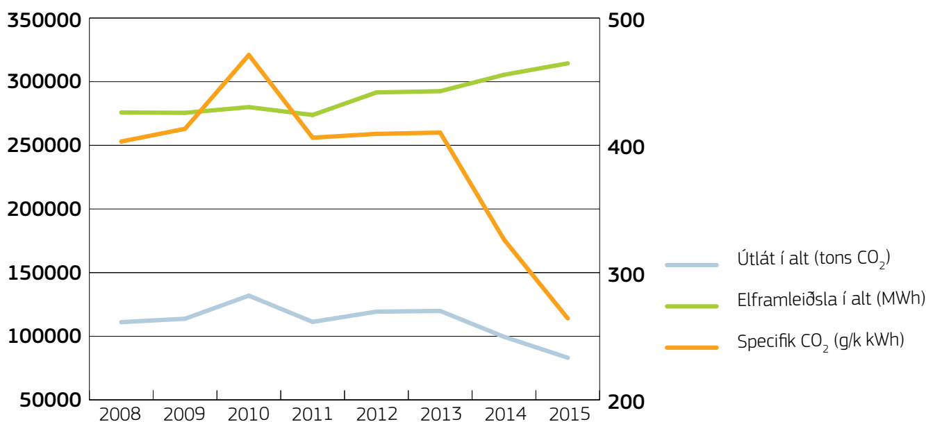
Mynd 5. Útlátið av CO 2 , elframleiðsan og specifik CO 2 frá 2008-2015.
