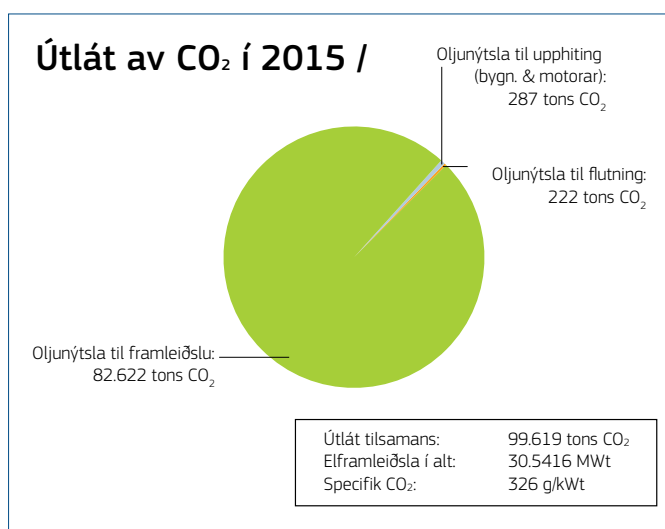
Mynd 4. Nøgdin av CO 2 -útláti í 2015.
